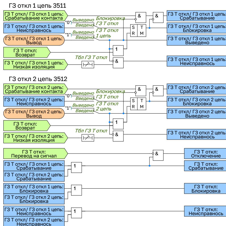
Рисунок 2.14 – Функциональная схема логики отключающей ступени ГЗ
