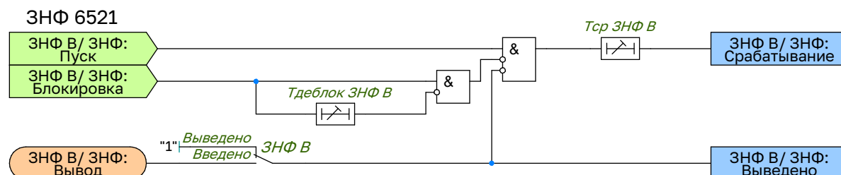
Рисунок 2.8 – Функциональная схема логики ЗНФ
