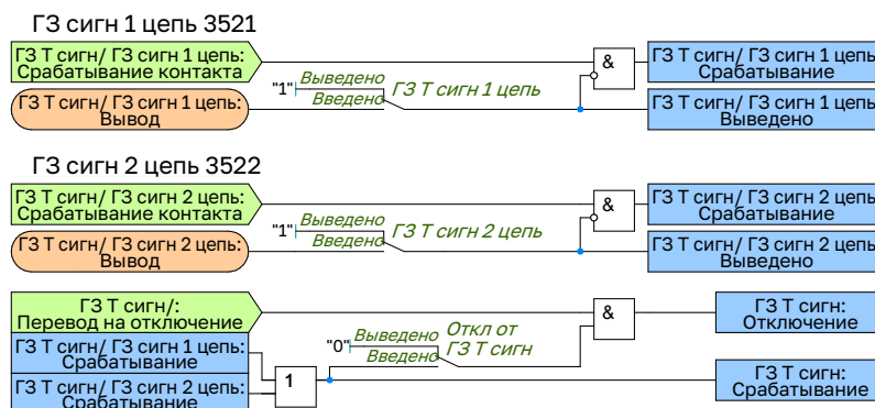
Рисунок 2.15 – Функциональная схема логики сигнальной ступени ГЗ
